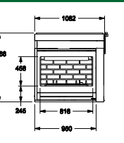
Pohľad spredu
