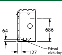
Pohľad sprava
