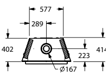
Pohľad zhora
