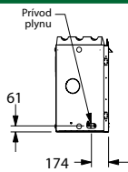
Pohľad zľava
