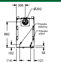
Pohľad zľava
