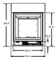
Pohľad spredu
