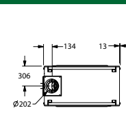
Pohľad zhora
