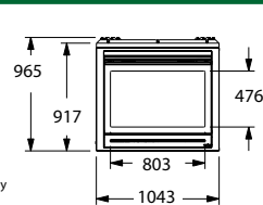
Pohľad spredu
