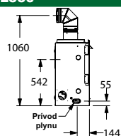
Pohľad zľava
