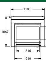
Pohľad spredu
