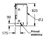
Pohľad sprava
